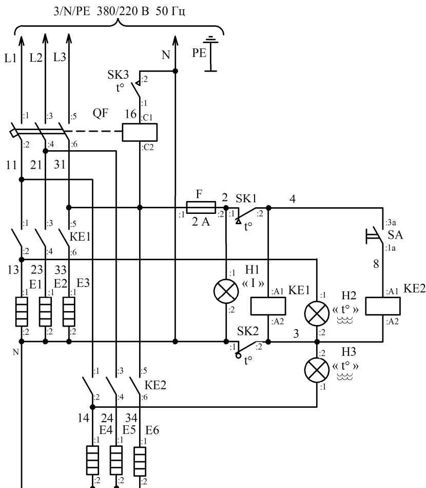
Рисунок 2 – Схема электрическая принципиальная водонагревателей ЭВА-450/15 и ЭВА-600/15
