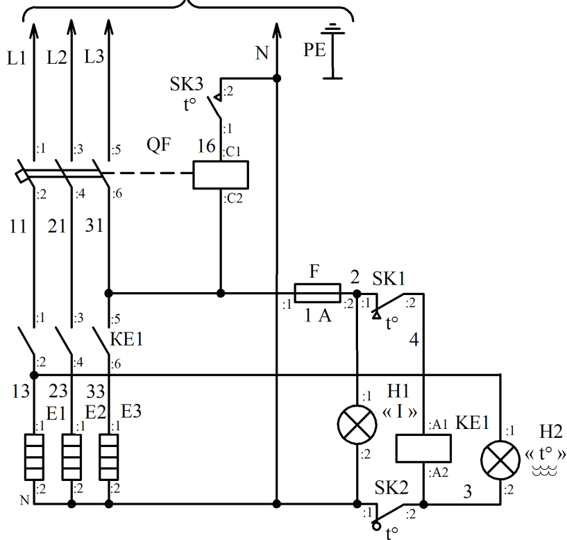
Рисунок 1 – Электроволоннагреватель аккумуляторный с термоизоляцией ЭВА. 3/Н/РЕ 380/220 В 50 Гц
