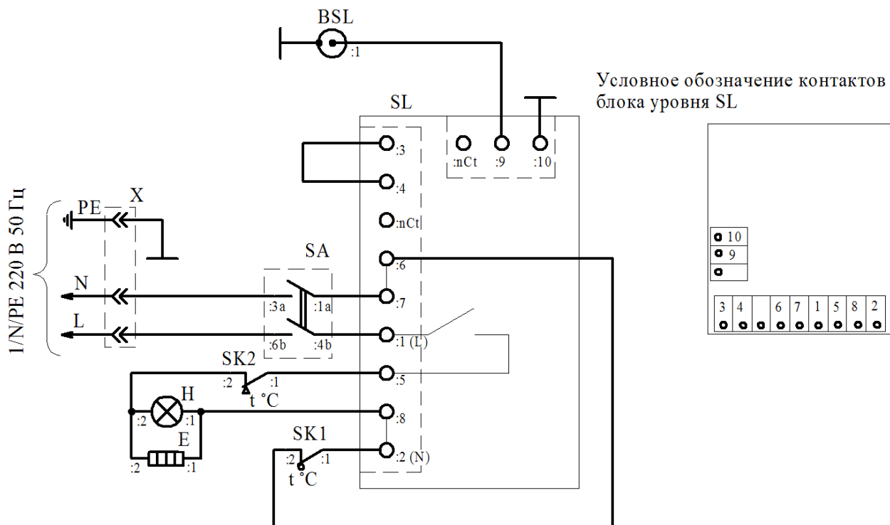
Рисунок 3 Схема электрическая принципиальная водонагревателей ЭВАО-10-01 и ЭВАО-15-01
