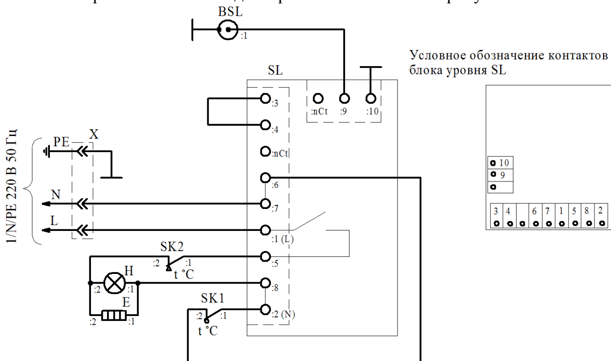
Рисунок 2 Схема электрическая принципиальная водонагревателей ЭВАО-10 и ЭВАО-15
