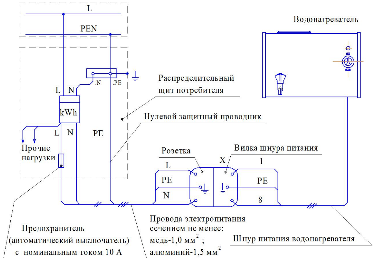
Рисунок 5 – Схема подключения водонагревателя
