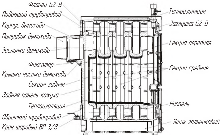
Рис. 2.2. Устройство котла. Вид сбоку в разрезе
