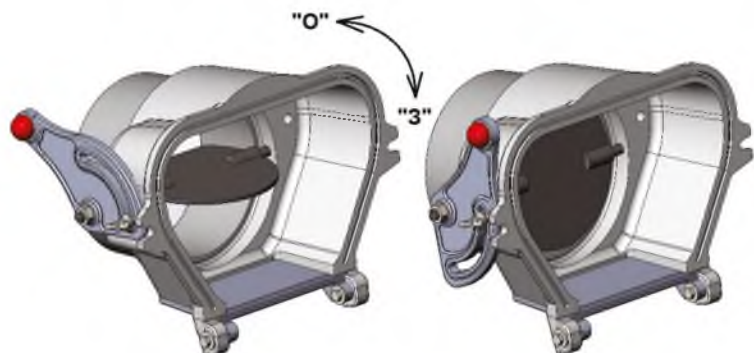
Рис.5 Шиберная заслонка
