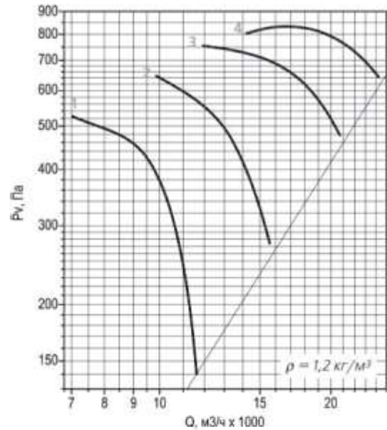
Аэродинамическая характеристика вентилятора ВО 30-160 № 7,1
