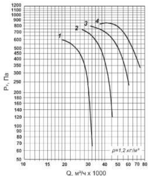
Аэродинамическая характеристика вентилятора ВО 30-160 № 11,2
