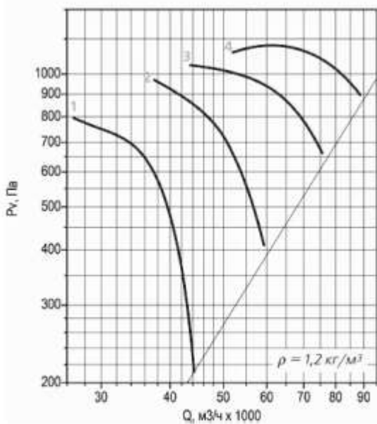
Аэродинамическая характеристика вентилятора ВО 30-160 № 12,5
