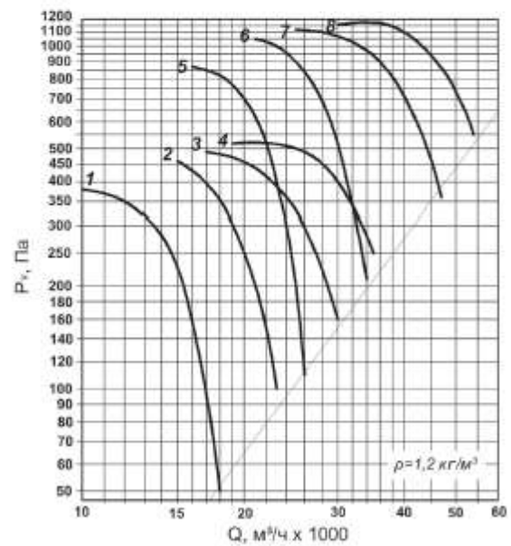
Аэродинамическая характеристика вентилятора ВО 30-160 № 9
