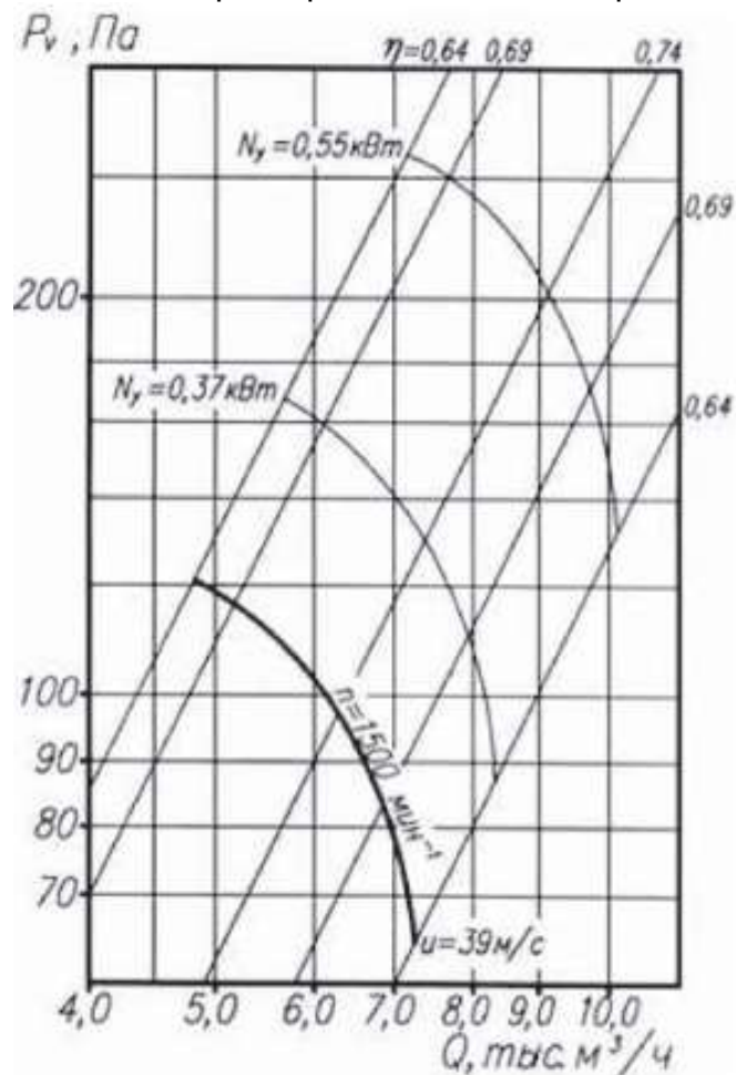
Аэродинамическая характеристика вентилятора ВО 06-300 №5
