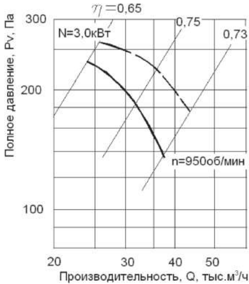
Аэродинамическая характеристика вентилятора В0 06-300 №10
