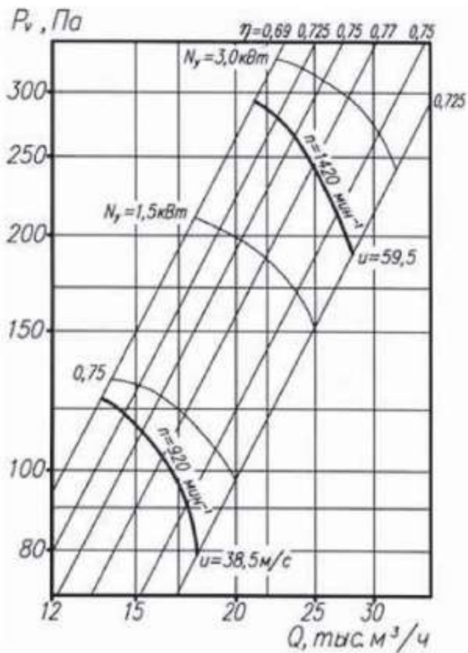
Аэродинамическая характеристика вентилятора ВО 06-300 №8
