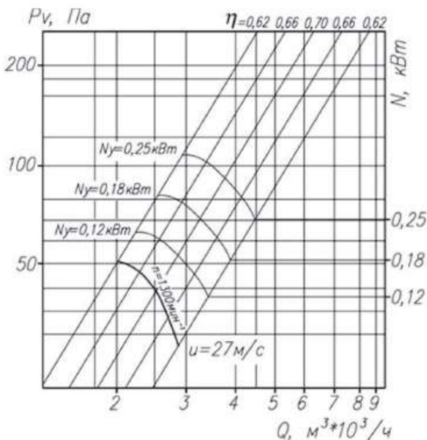
Аэродинамическая характеристика вентилятора ВО 06-300 №3,15
