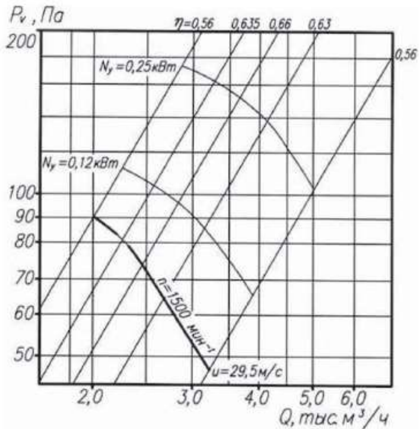
Аэродинамическая характеристика вентилятора ВО 06-300 №4
