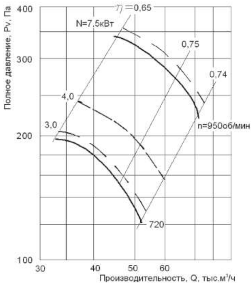
Аэродинамическая характеристика вентилятора В0 06-300 №12,5
