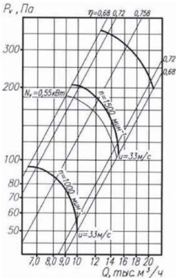
Аэродинамическая характеристика вентилятора ВО 06-300 №6,3
