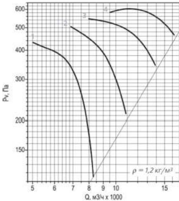
Аэродинамическая характеристика вентиляторов ВО 30-160 № 6,3
