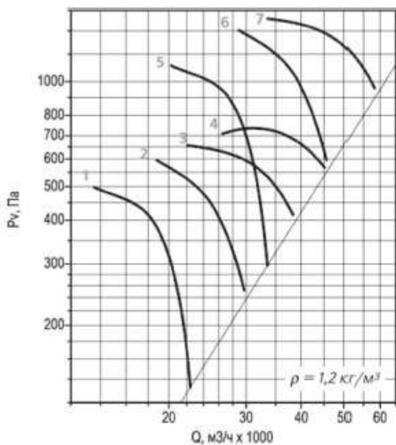
Аэродинамическая характеристика вентилятора ВО 30-160 № 10
