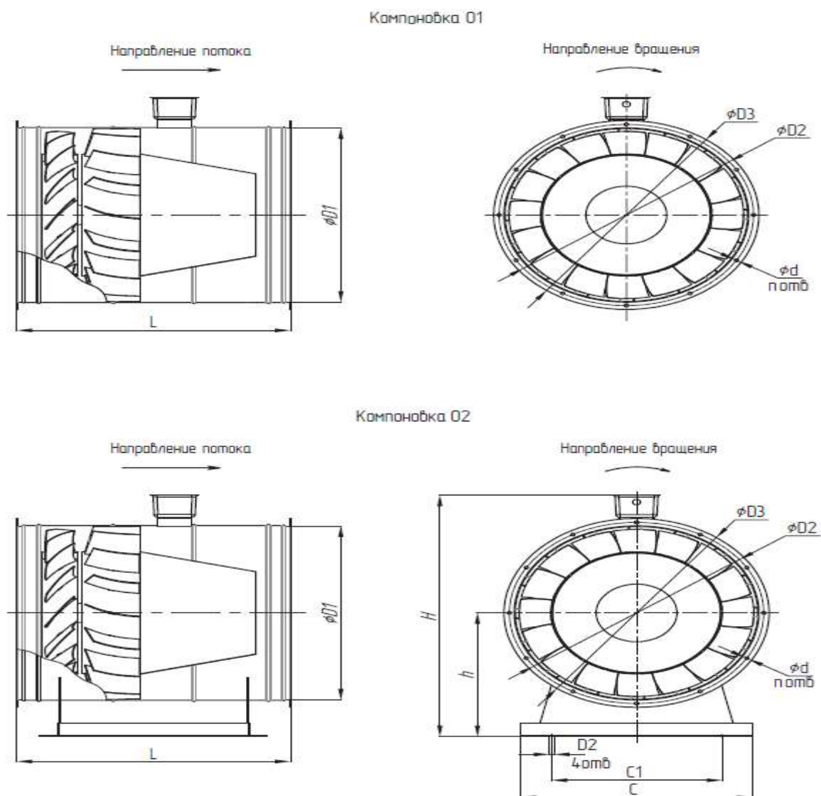
Рис.1. Габаритно присоединительные размеры ВО 30-160
