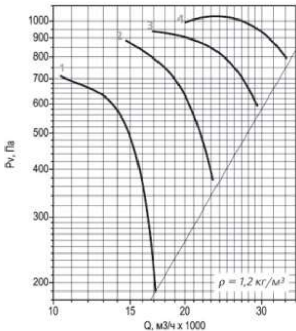
Аэродинамическая характеристика вентилятора ВО 30-160 № 8
