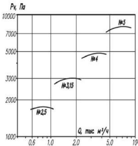
Аэродинамическая характеристика вентиляторов ВР 12-26-2
