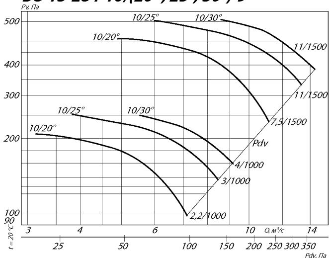
ВО 13-284-10/(20°, 25°, 30°)-9
