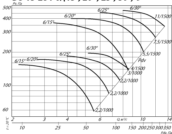
ВО 13-284-6/(15°, 20°, 25°, 30°)-9
