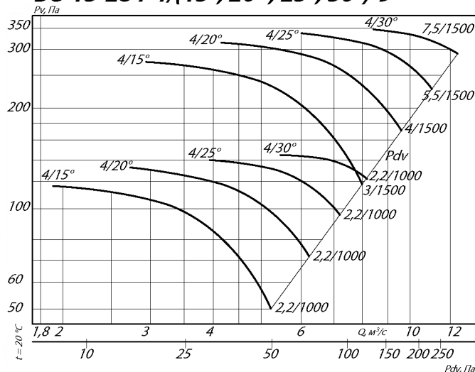
ВО 13-284-4/(15°, 20°, 25°, 30°)-9
