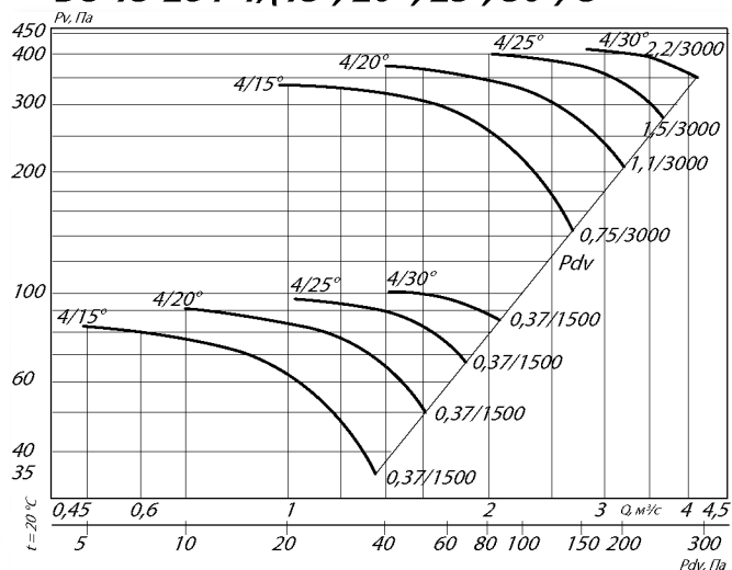
ВО 13-284-4/(15°, 20°, 25°, 30°)-5
