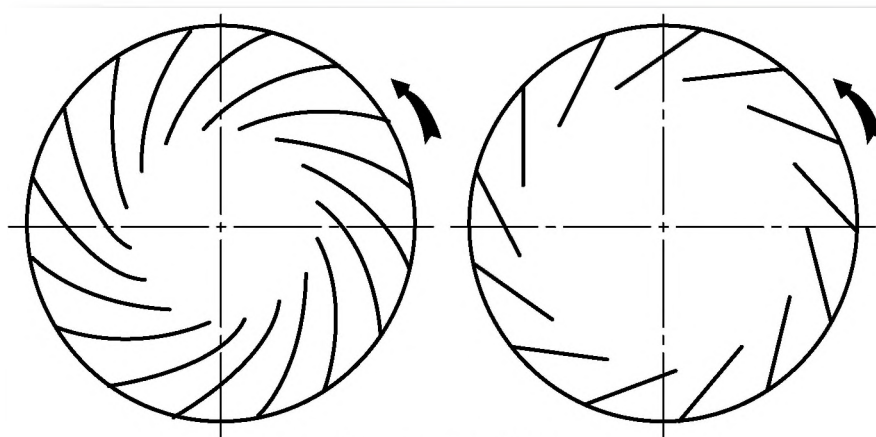
Назад загнутые лопатки
