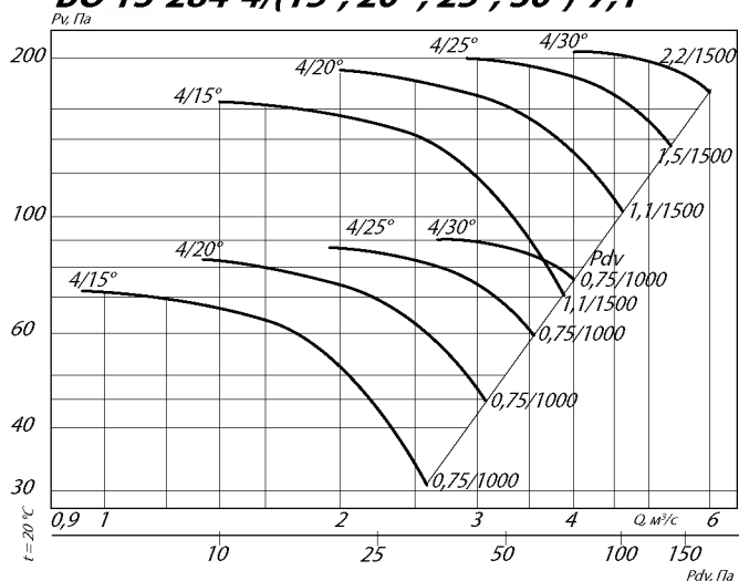
ВО 13-284-4/(15°, 20°, 25°, 30°)-7,1
