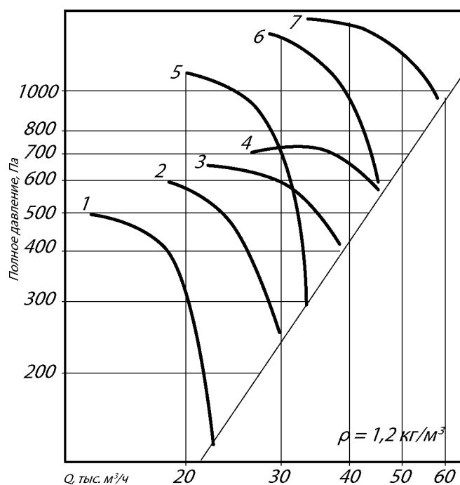
ВО 30-160-10
