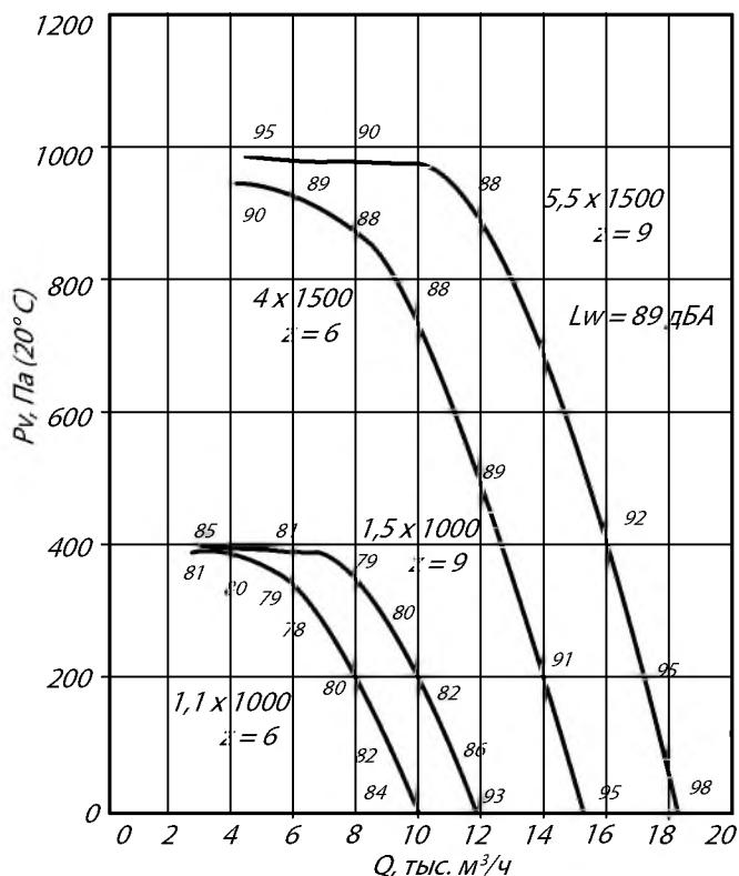
ВКРФ 6,3
