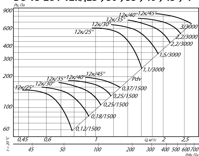
ВО 13-284-12к/(25°, 30°, 35°, 40°, 45°)-4
