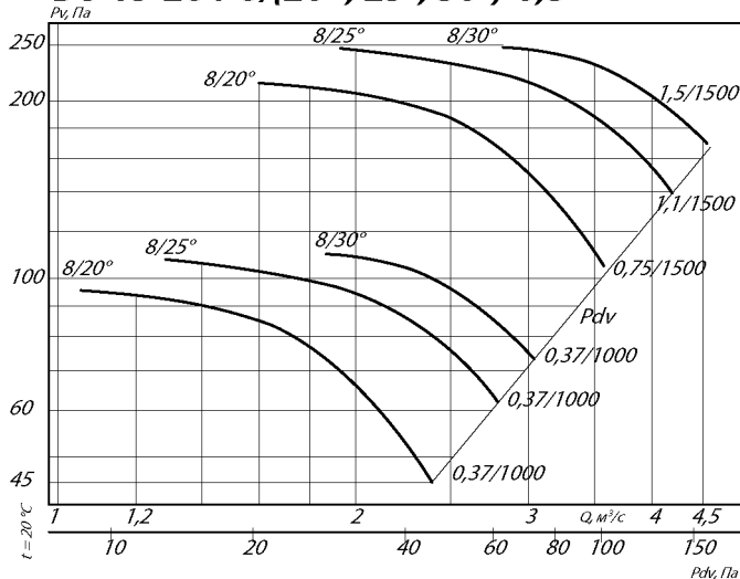
ВО 13-284-8/(20°, 25°, 30°)-6,3
