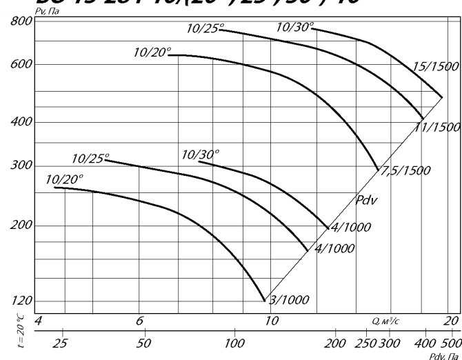
ВО 13-284-10/(20°, 25°, 30°)-10
