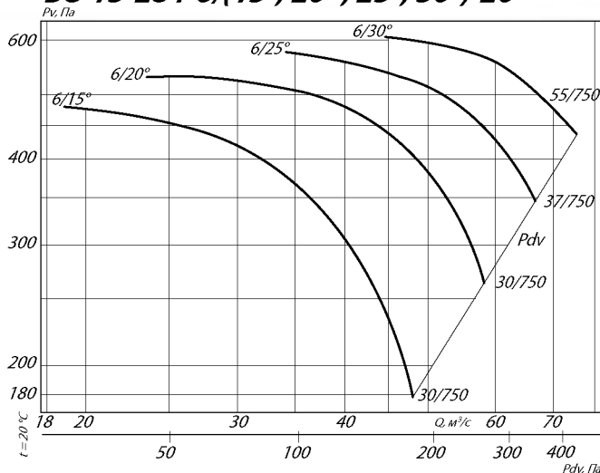
ВО 13-284-6/(15°, 20°, 25°, 30°)-20
