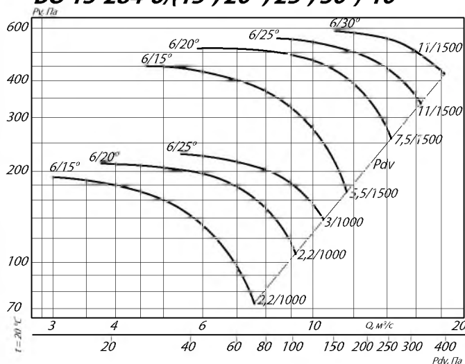
ВО 13-284-6/(15°, 20°, 25°, 30°)-10
