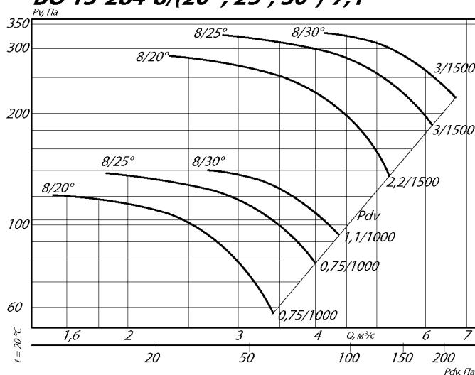
ВО 13-284-8/(20°, 25°, 30°)-7,1
