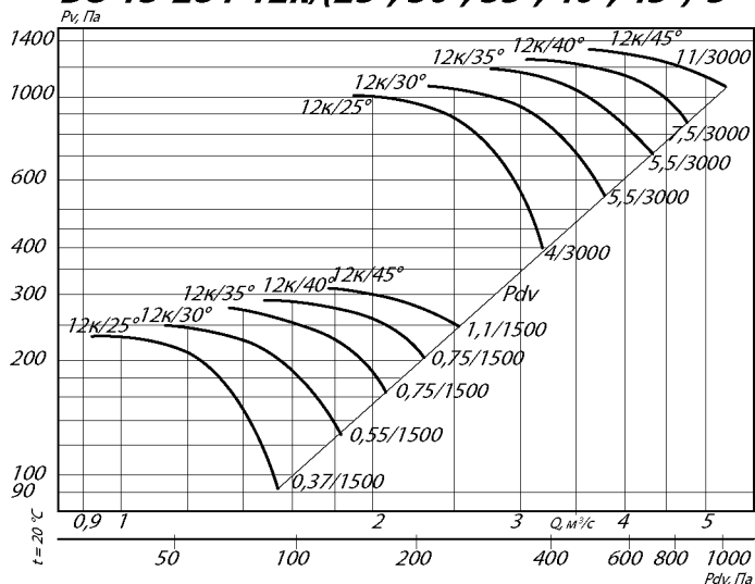
ВО 13-284-12к/(25°, 30°, 35°, 40°, 45°)-5
