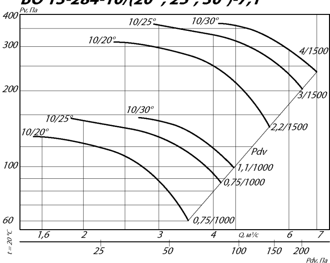
ВО 13-284-10/(20°, 25°, 30°)-7,1
