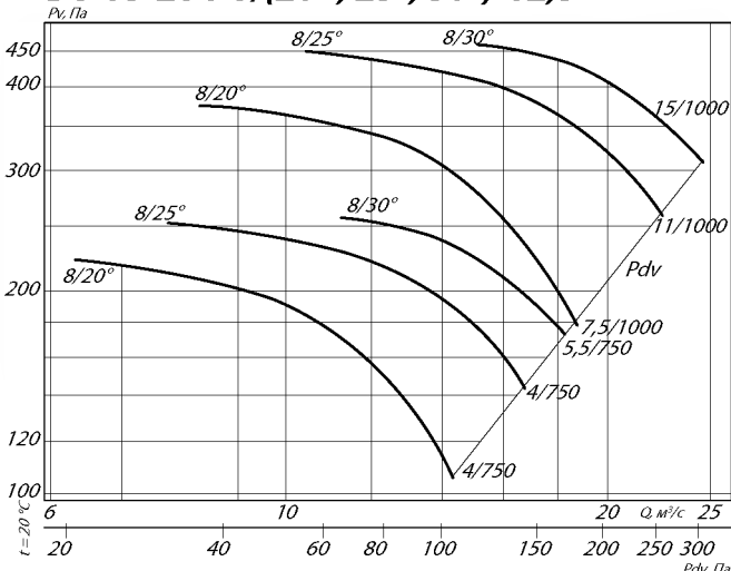
ВО 13-284-8/(20°, 25°, 30°)-12,5
