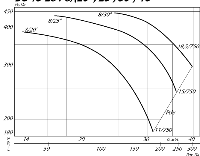
ВО 13-284-8/(20°, 25°, 30°)-16
