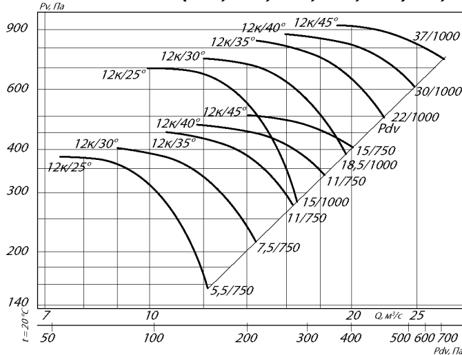
ВО 13-284-12к/(25°, 30°, 35°, 40°, 45°)-12,5
