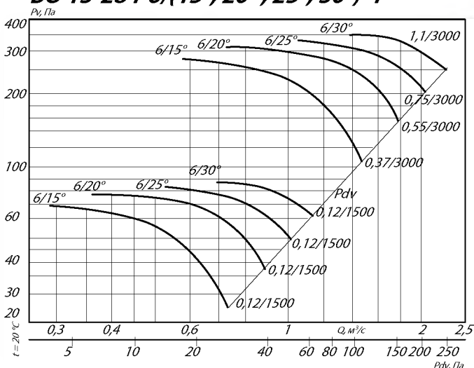
ВО 13-284-6/(15°, 20°, 25°, 30°)-4
