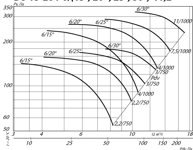
ВО 13-284-6/(15°, 20°, 25°, 30°)-11,2
