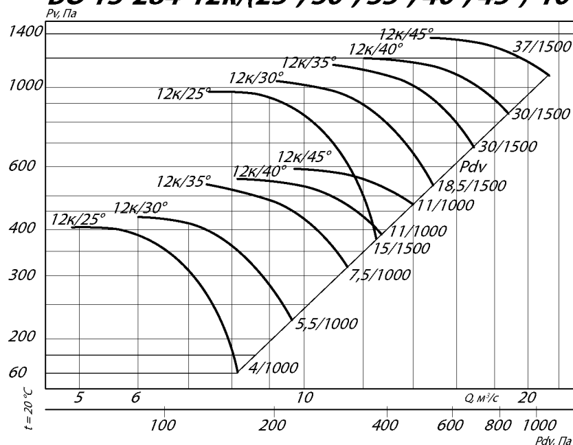
ВО 13-284-12к/(25°, 30°, 35°, 40°, 45°)-10
