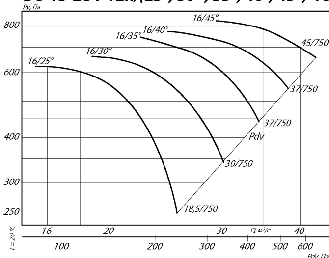
ВО 13-284-12к/(25°, 30°, 35°, 40°, 45°)-16
