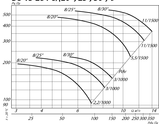
ВО 13-284-8/(20°, 25°, 30°)-9
