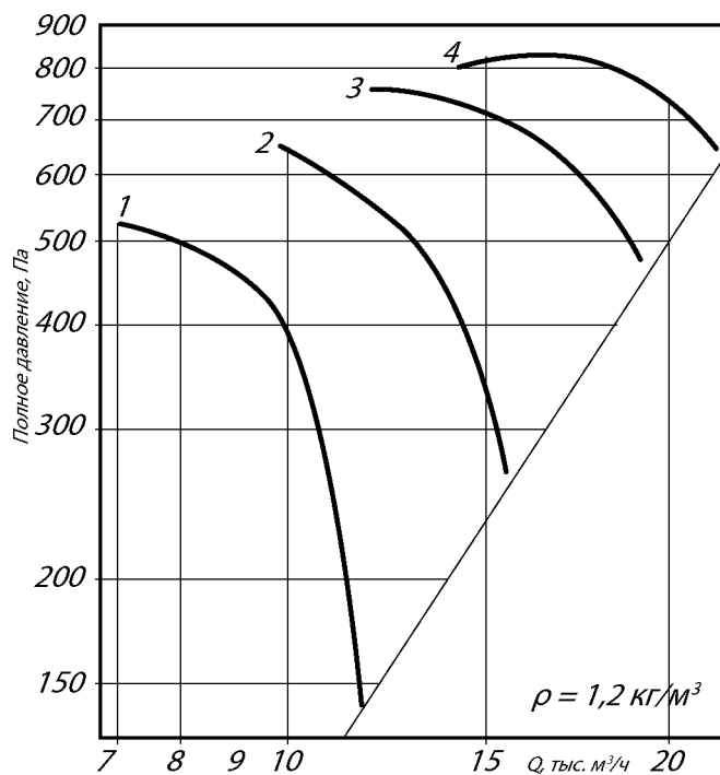
ВО 30-160-7,1
