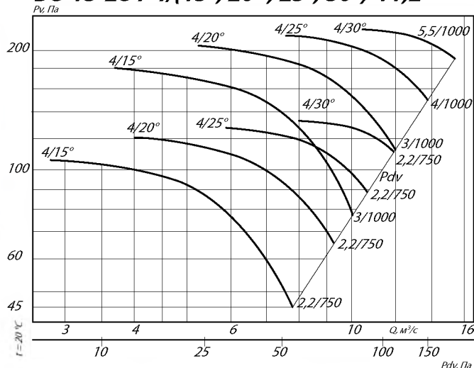
ВО 13-284-4/(15°, 20°, 25°, 30°)-11,2
