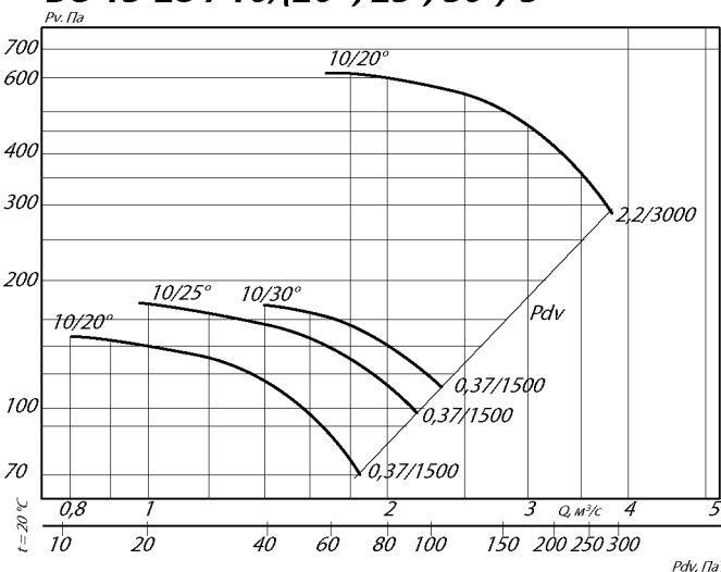
ВО 13-284-10/(20°, 25°, 30°)-5
