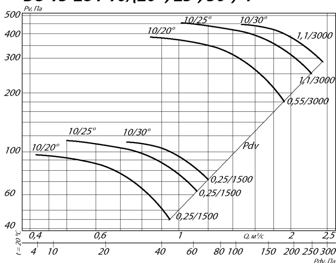
ВО 13-284-10/(20°, 25°, 30°)-4
