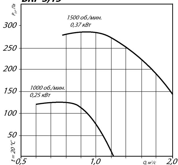
ВКР 3,15
