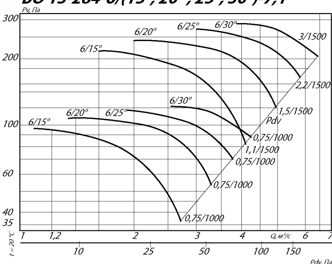
ВО 13-284-6/(15°, 20°, 25°, 30°)-7,1
