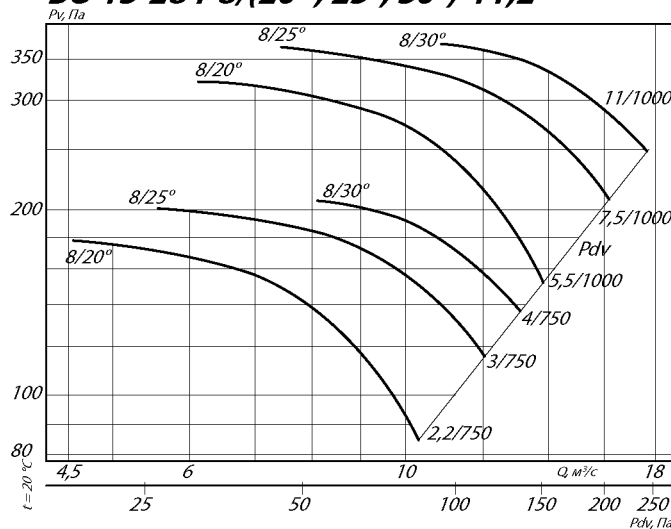
ВО 13-284-8/(20°, 25°, 30°)-11,2
