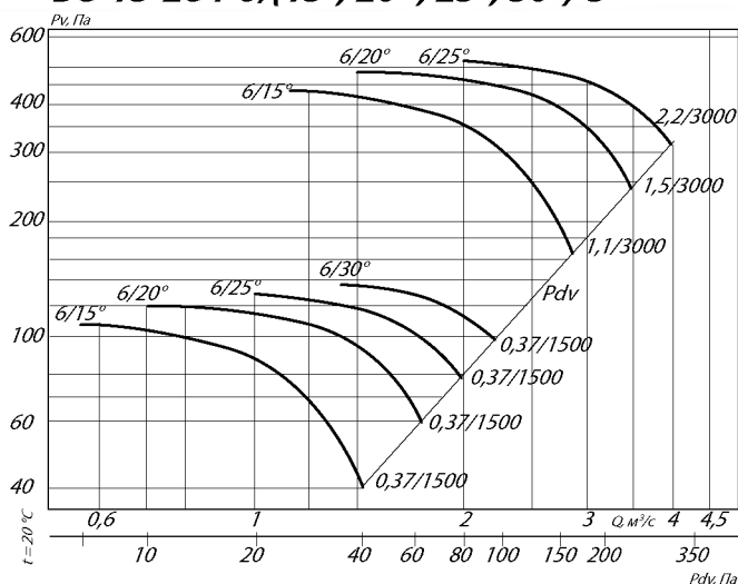
ВО 13-284-6/(15°, 20°, 25°, 30°)-5
