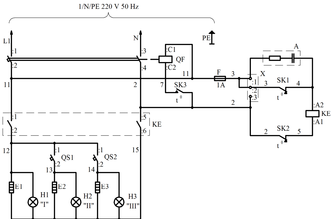
Рисунок 3 - Схема электрическая принципиальная ЭВО-4,8-01.
