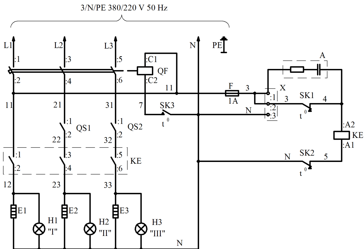
Рисунок 2 - Схема электрическая принципиальная ЭВО-15, ЭВО-9, ЭВО-4,8.
