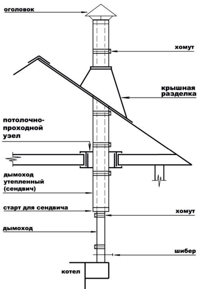
Рис. 3 — Схема дымохода
