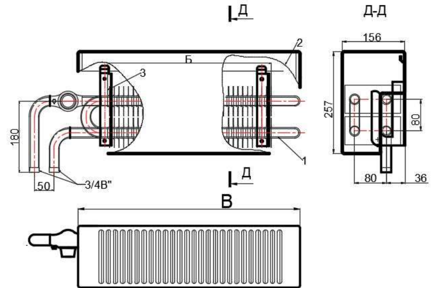
Рис. 2. Конвектор «Универсал» Мини КСК 20 СР-2 К v ниж/лев. (концевой для левого нижнего присоединения с термостатом КТК П-2.1, оснащённым воздухоотводчиком):
