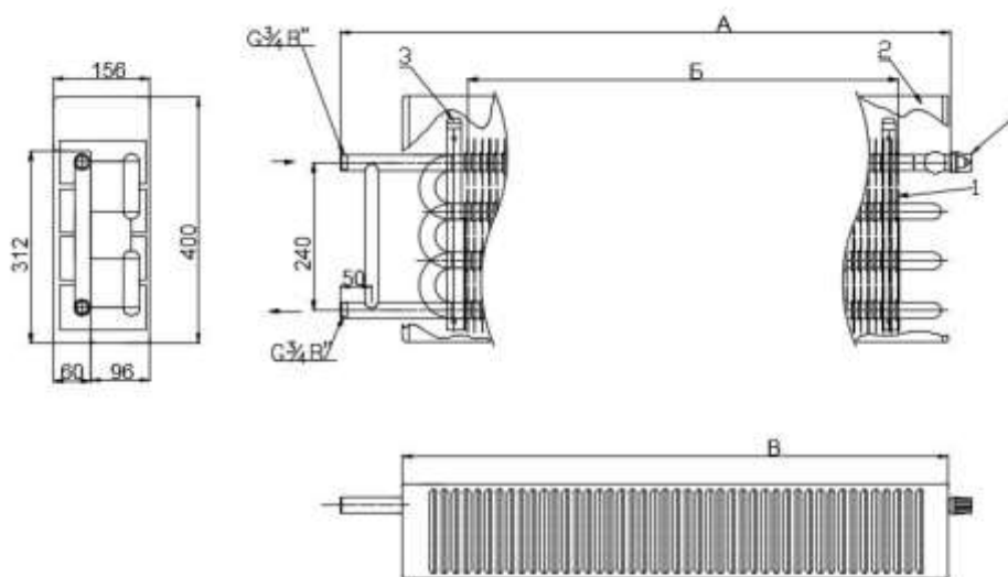
Рис. 1. Конвектор «Универсал» КСК 20 Супер СТ-1 К в лев. ЗУ (Конвектор концевой для однотрубной системы левого присоединения с розливом теплоносителя «сверху – вниз» и замыкающим участком, а так же термостатом КТК У-1):
