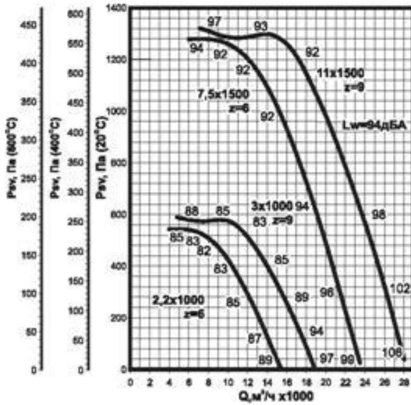
Аэродинамическая характеристика вентилятора ВКРС ДУ №7,1
