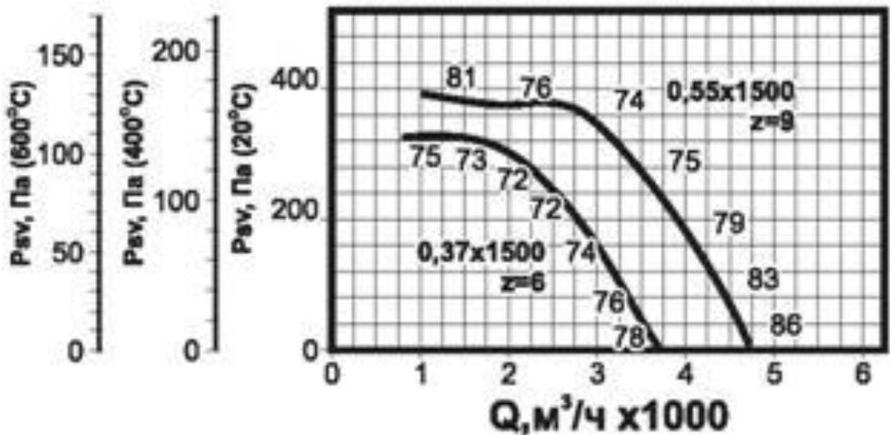
Аэродинамическая характеристика вентилятора ВКРС ДУ №4
