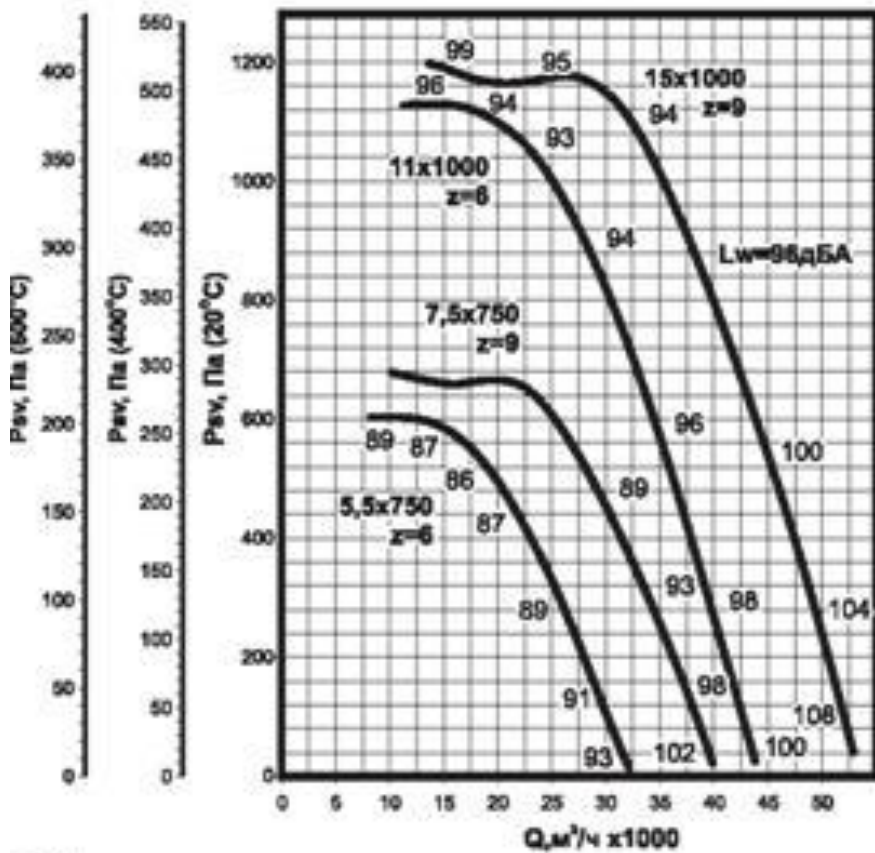
Аэродинамическая характеристика вентилятора ВКРС ДУ №10
