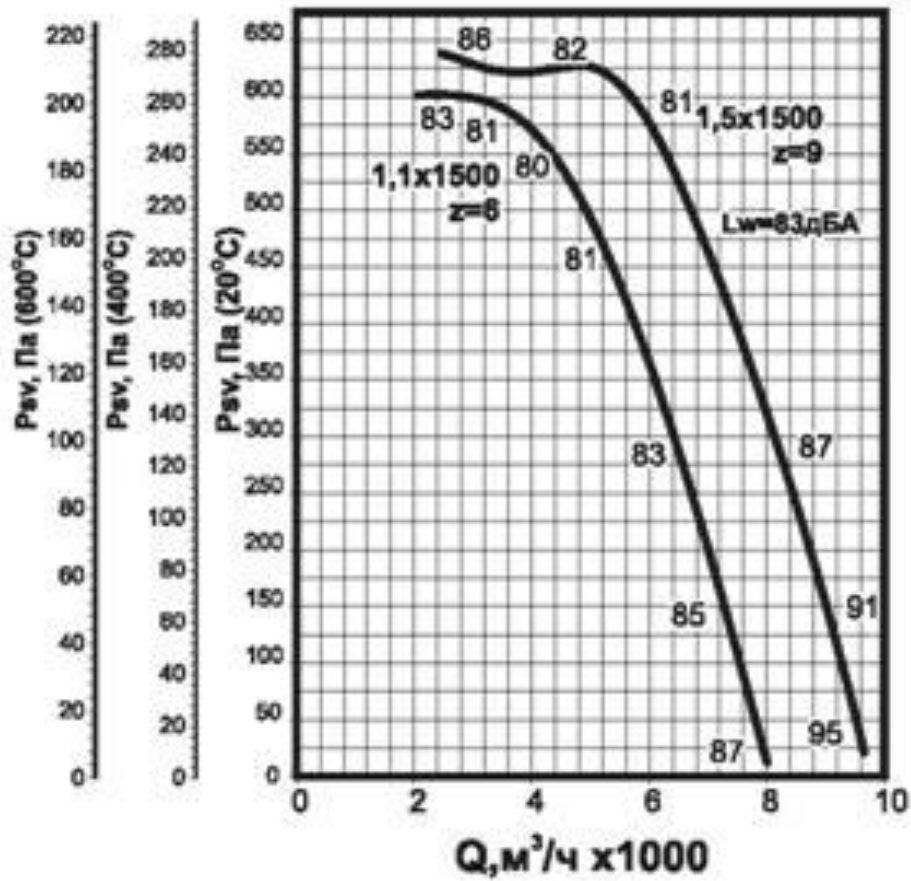
Аэродинамическая характеристика вентилятора ВКРС ДУ №5
