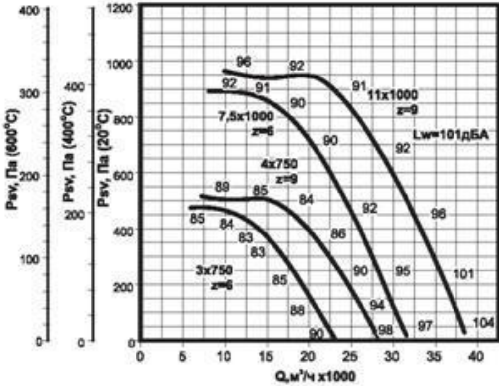
Аэродинамическая характеристика вентилятора ВКРС ДУ №9
