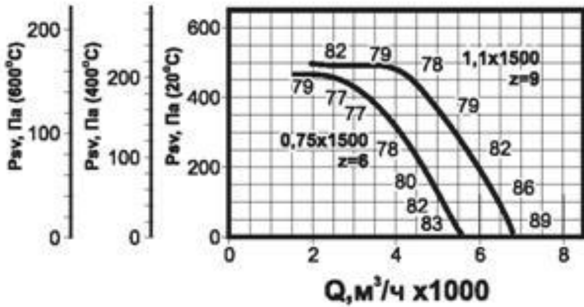
Аэродинамическая характеристика вентилятора ВКРС ДУ №4,5
