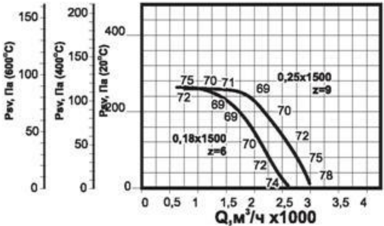
Аэродинамическая характеристика вентилятора ВКР ДУ №3,55
