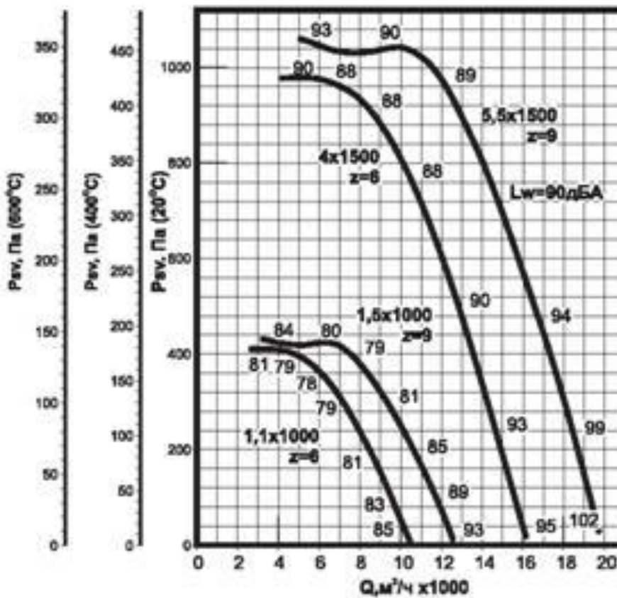
Аэродинамическая характеристика вентилятора ВКРС ДУ №6,3
