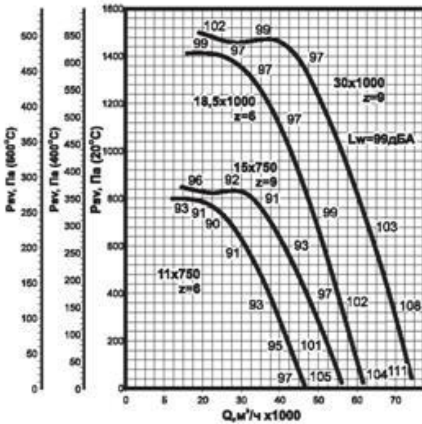
Аэродинамическая характеристика вентилятора ВКРС ДУ №11,2
