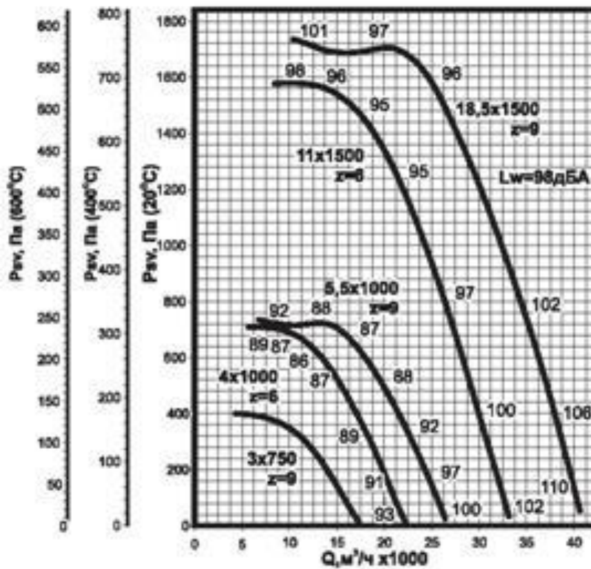
Аэродинамическая характеристика вентилятора ВКРС ДУ №7,1
