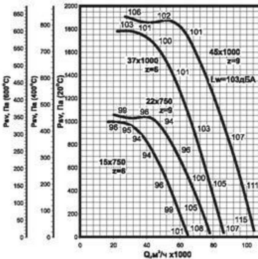
Аэродинамическая характеристика вентилятора ВКРС ДУ №12,5
