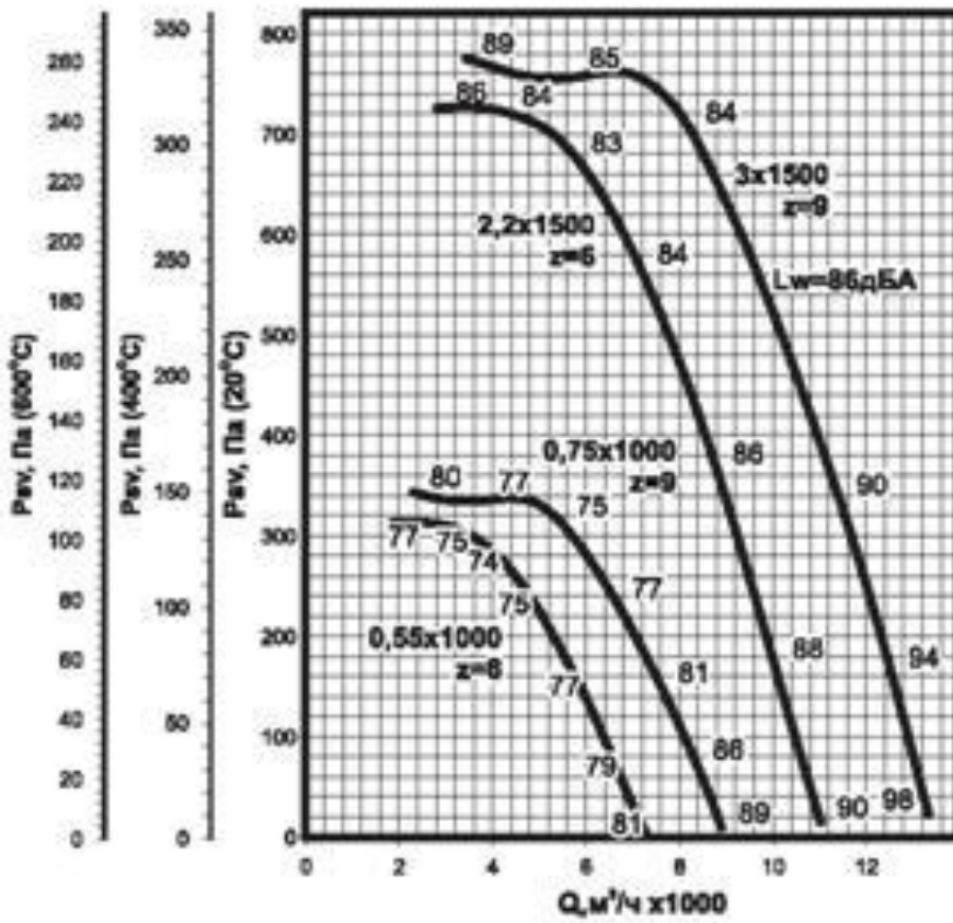
Аэродинамическая характеристика вентилятора ВКРС ДУ №5,6
