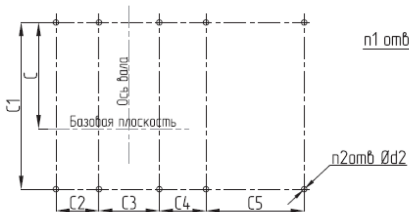
Схема расположения отверстий для крепления вентилятора ВР 80-75-8...12,5
