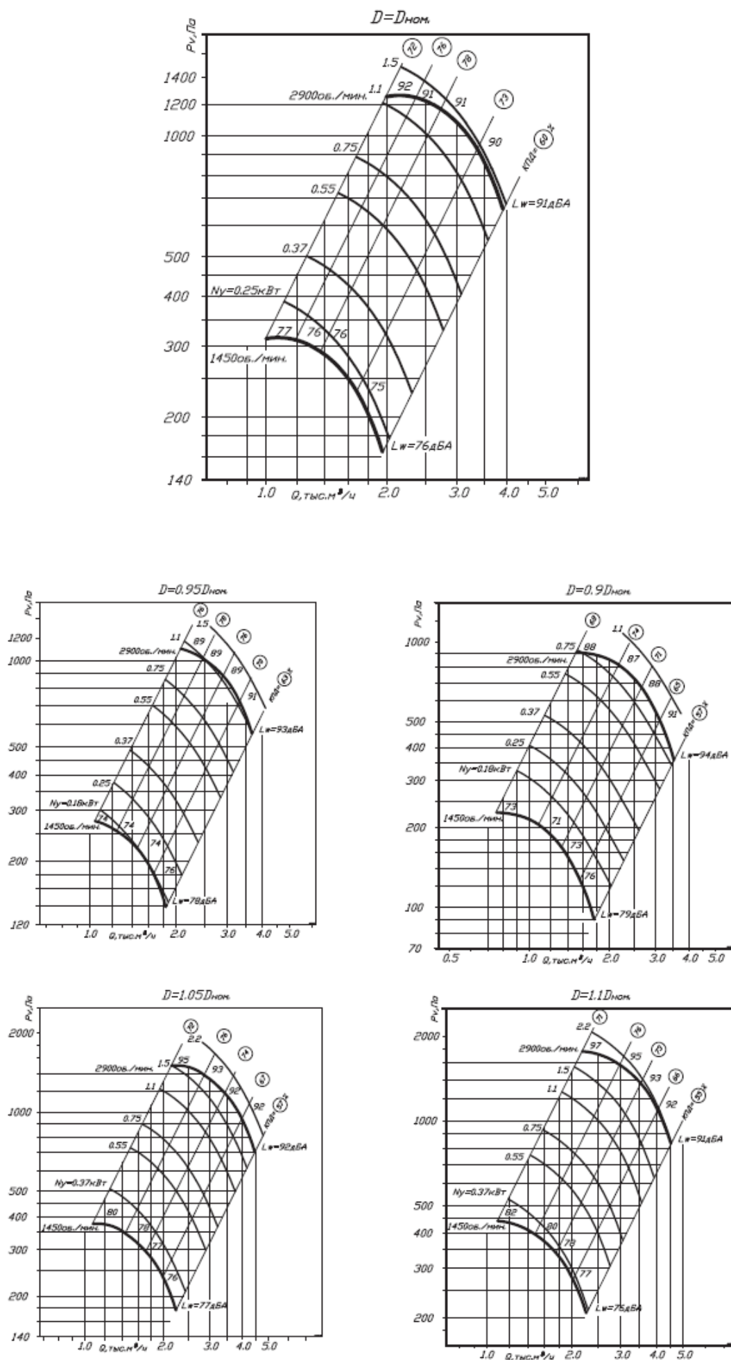
Аэродинамическая характеристика вентилятора ВР 80-75 №3,15 сх.1
