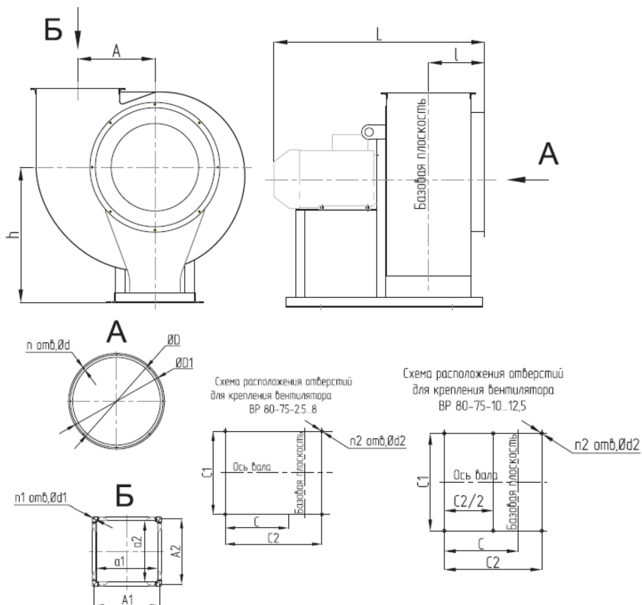
РИС. 1. Габаритные и присоединительные размеры вентиляторов ВР 80-75
