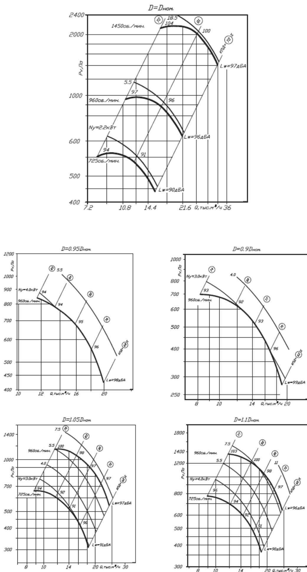
Аэродинамическая характеристика вентилятора ВР 80-75 №8 сх.1
