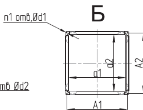
Выходной фланец
